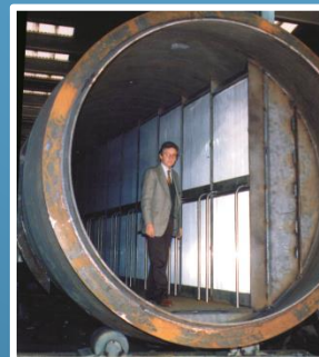
SLV TYPE - 130" # 150 LENGHT 21 m, 55 Ton
